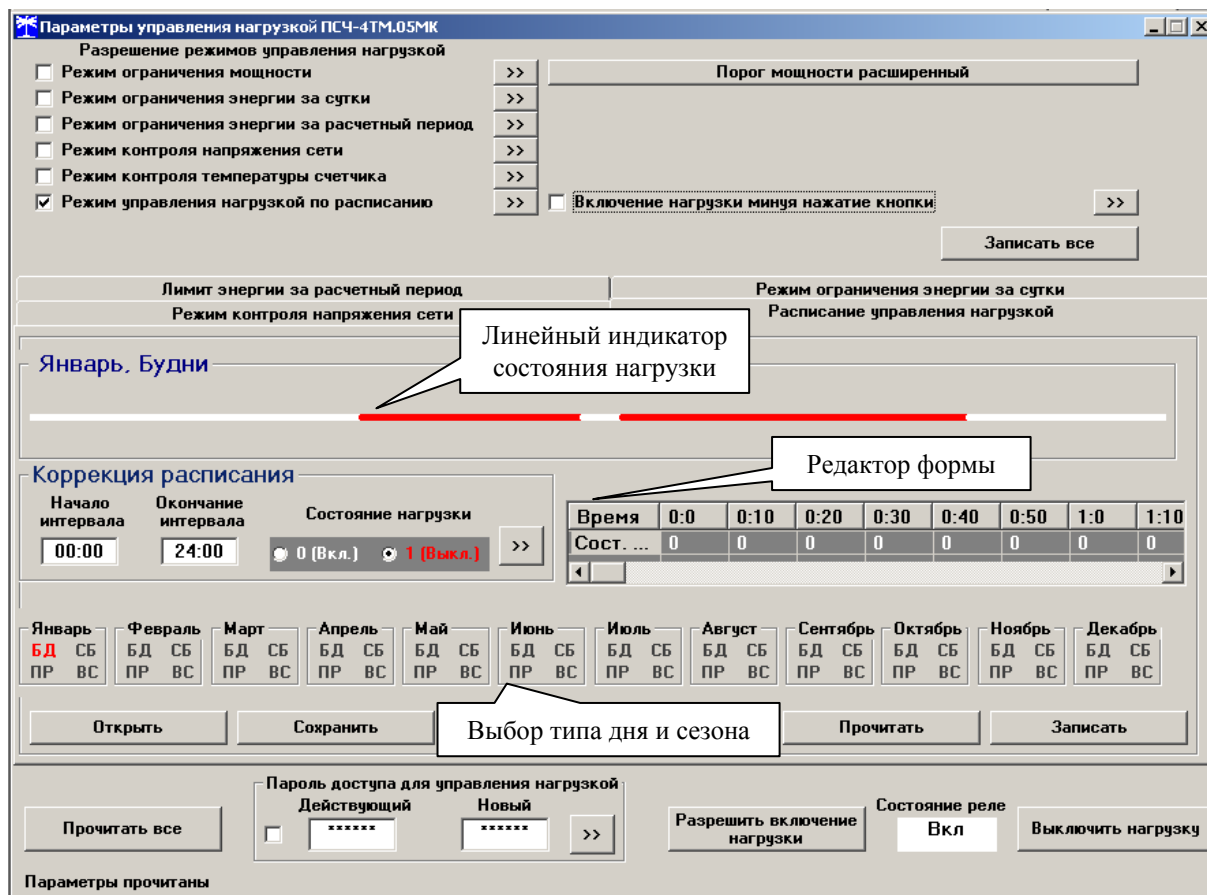
Рисунок 31 – Вкладка «Расписание управления нагрузкой»
