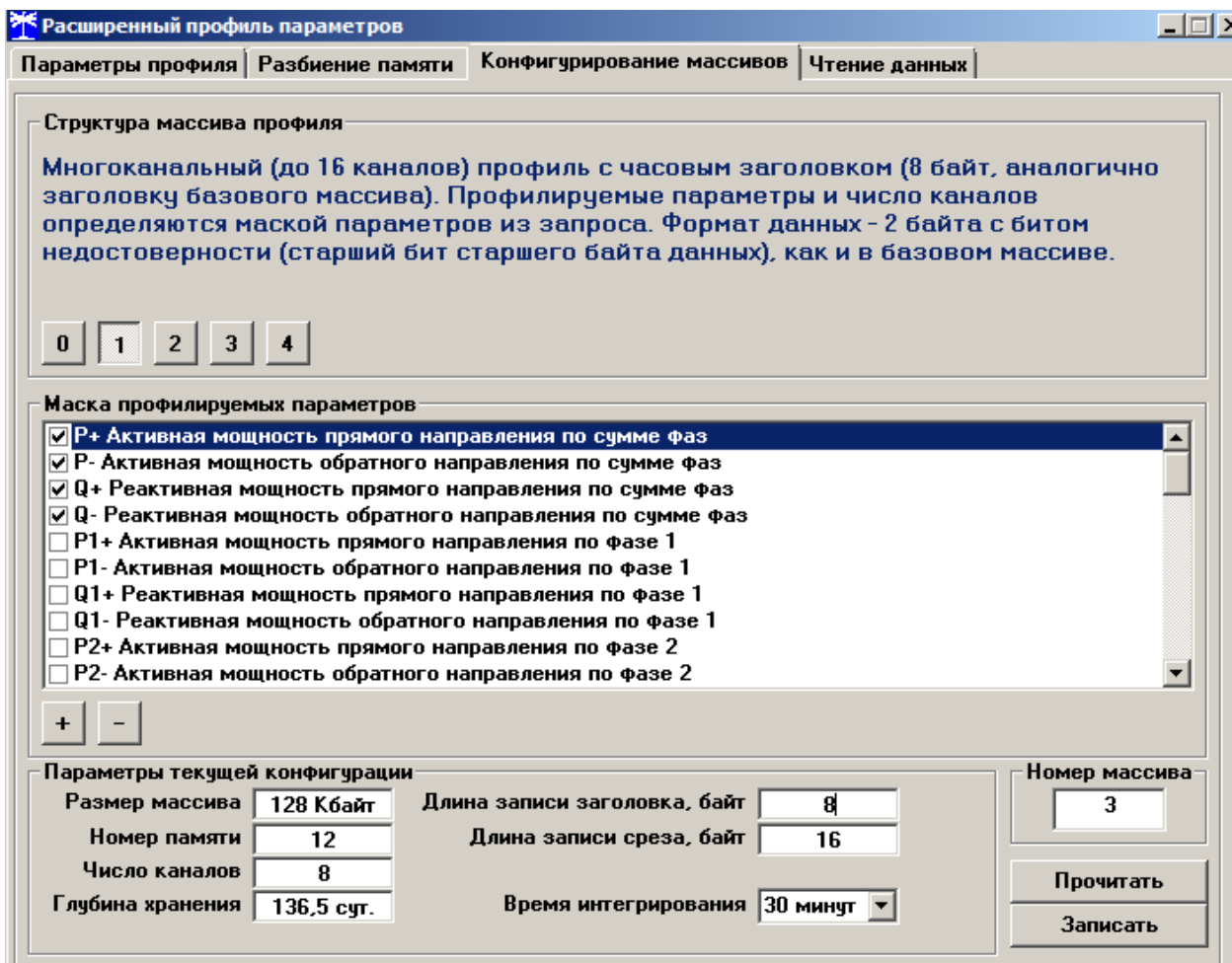
Рисунок 18 - Форма «Расширенный профиль параметров», вкладка «Конфигурирование массива»
