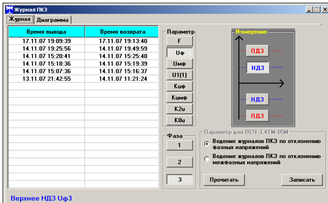
Рисунок 35 –Форма «Журналы ПКЭ» табличное представление
