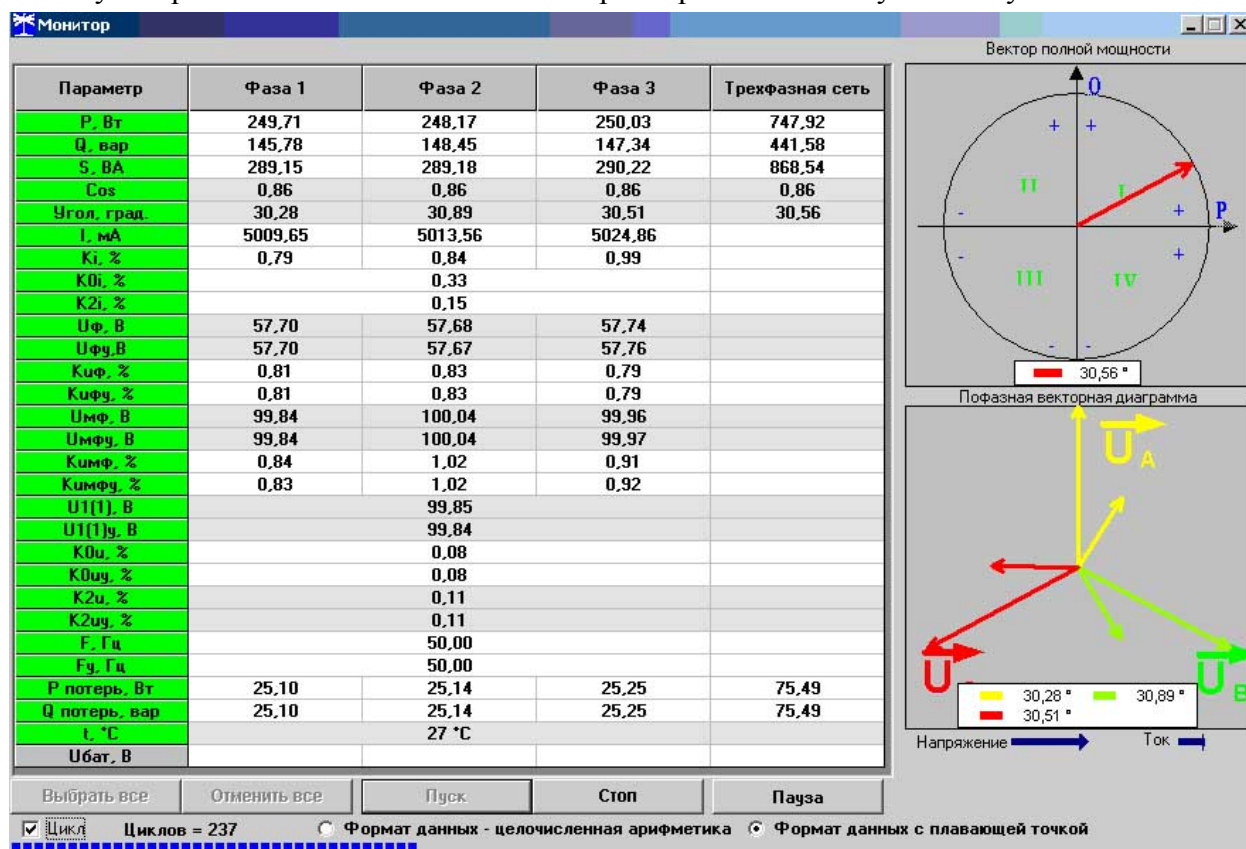
Рисунок 33 – Форма «Монитор»
