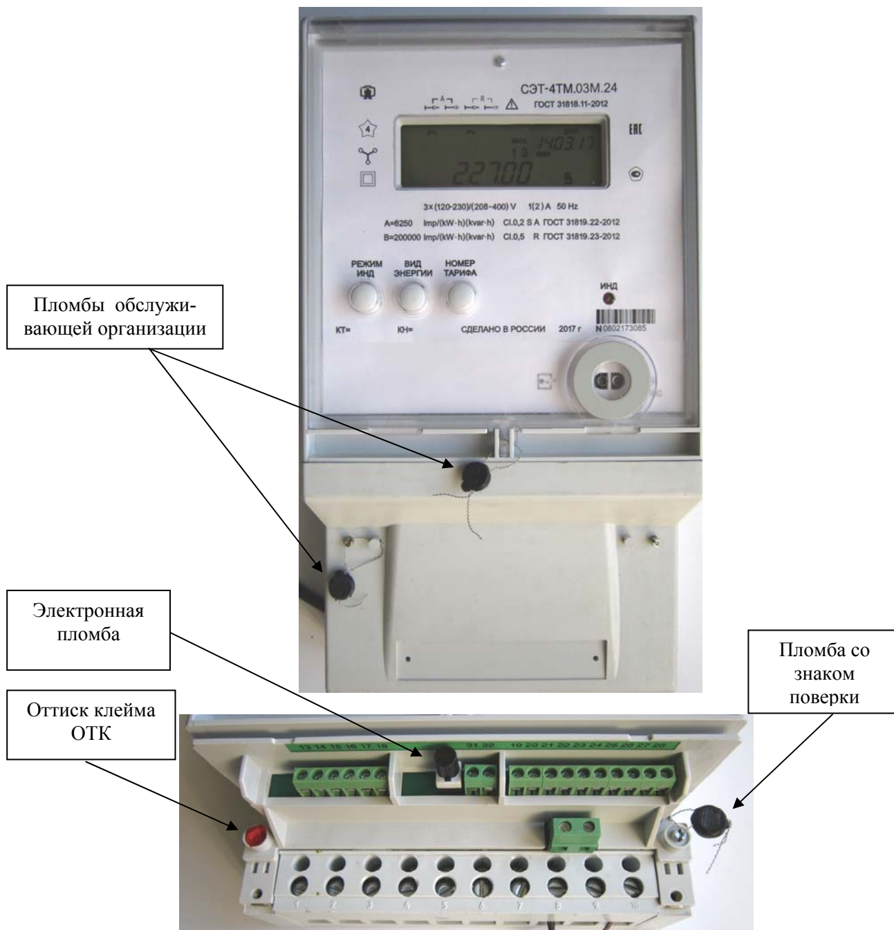
Рисунок 1 – Общий вид счетчика, схема пломбирования от несанкционированного доступа, обозначение места нанесения знака поверки
